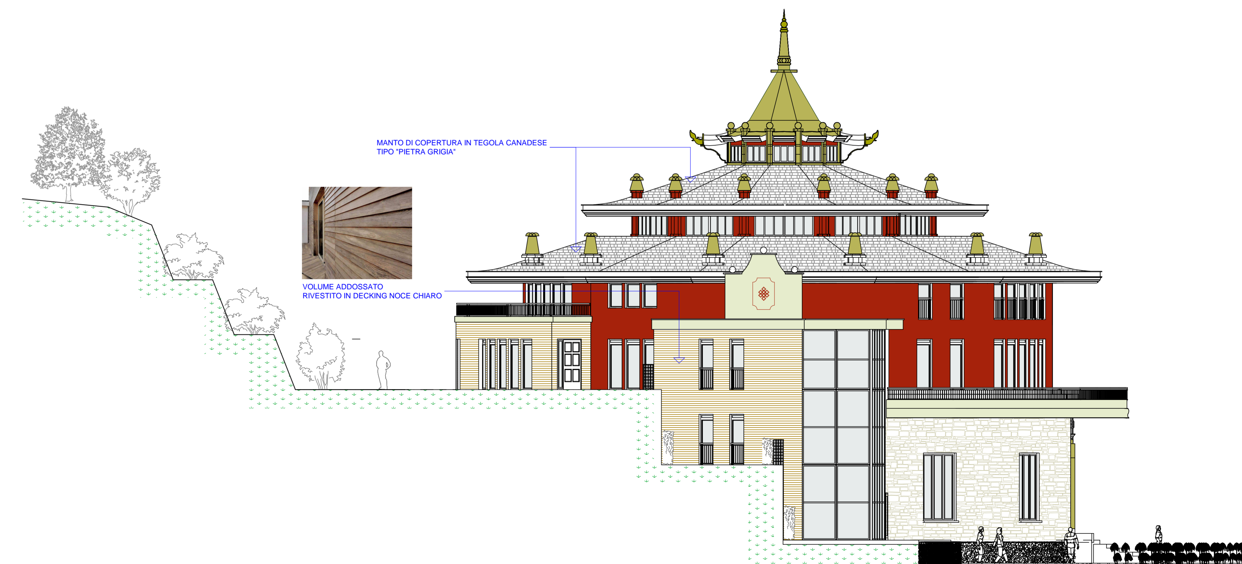
PROSPETTO OVEST
